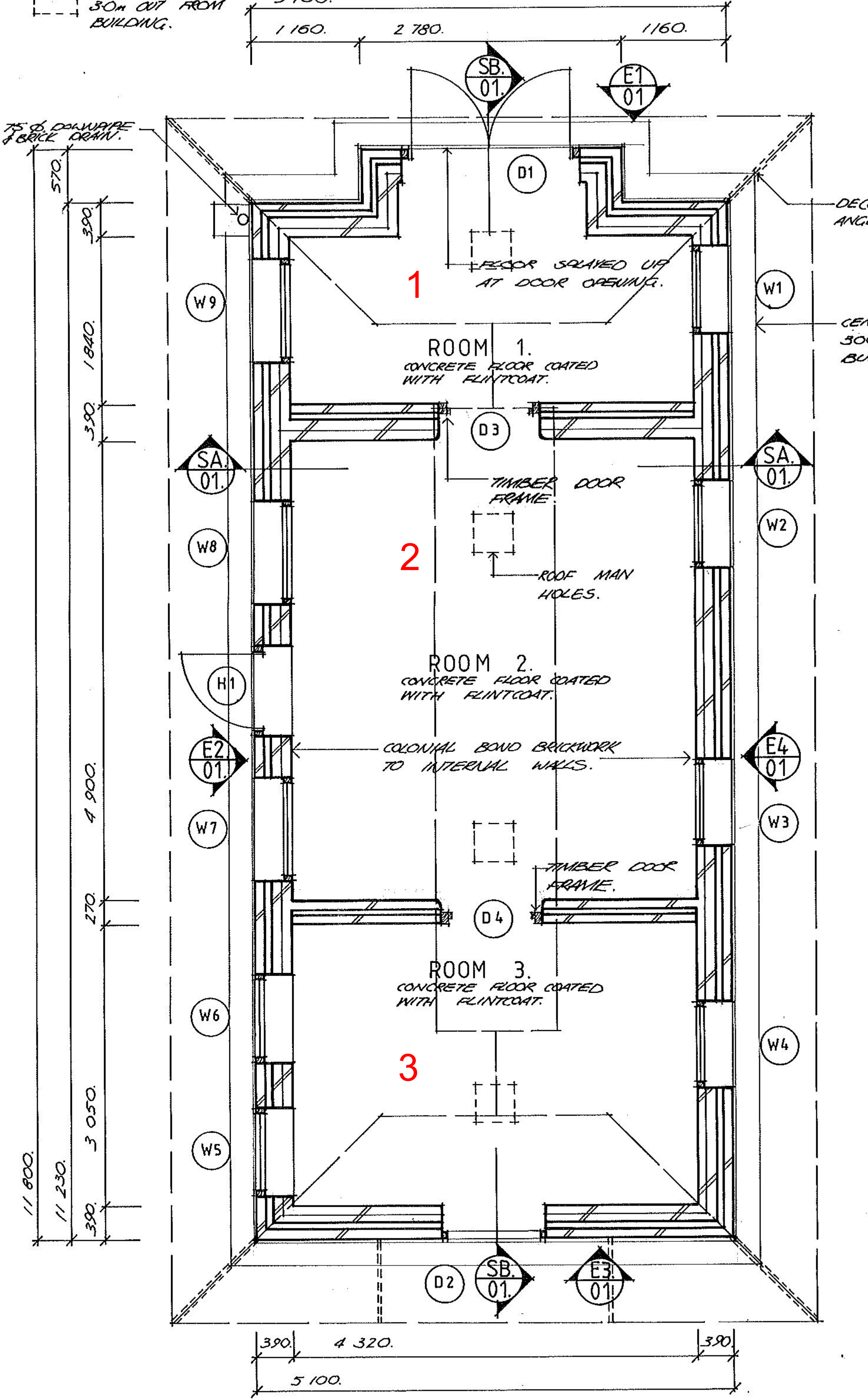
PLAN. 1:50.
